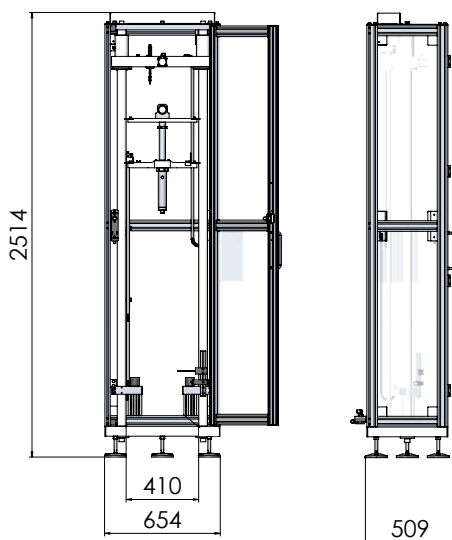
DW750 - Dimensions
