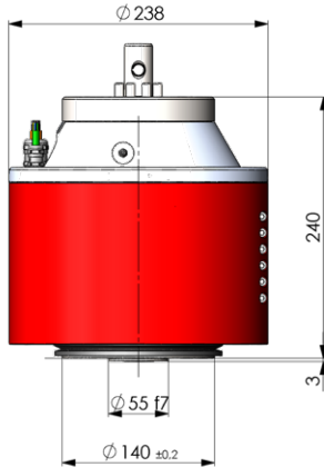
BV170 - Dimensions
